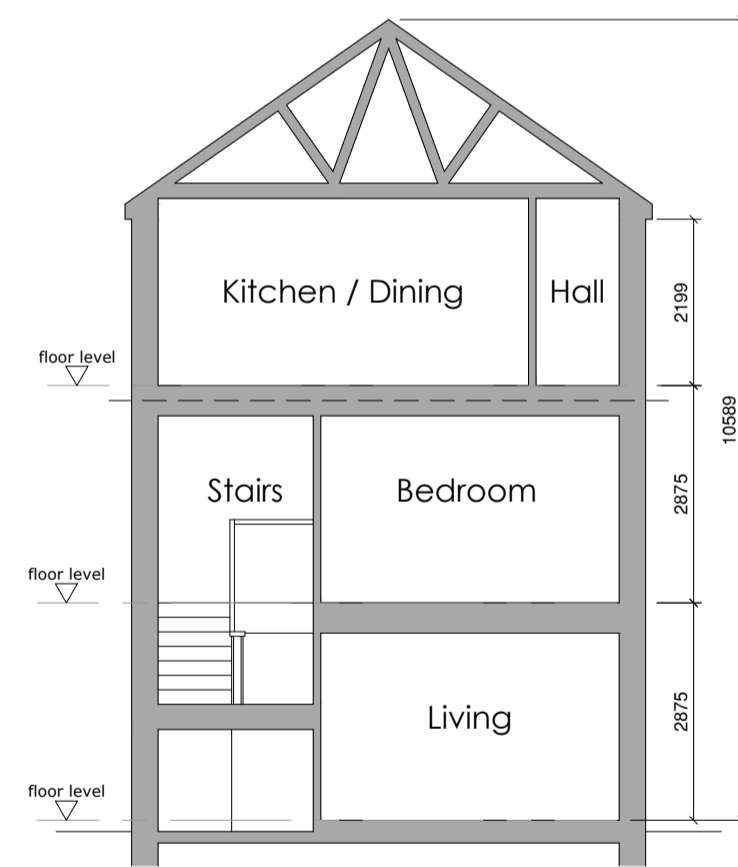
Section A-A
